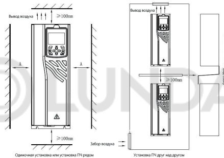
Рис. 3.1 Схема установки преобразователя частоты
